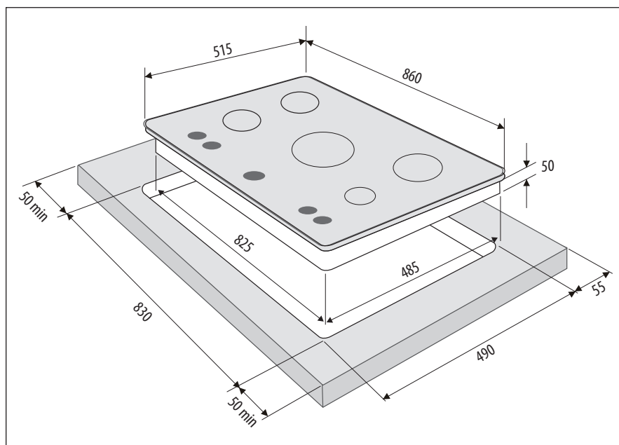
Схема встраивания варочной поверхности NOVANTA 90
